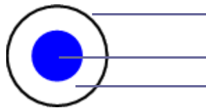
单选框按钮
