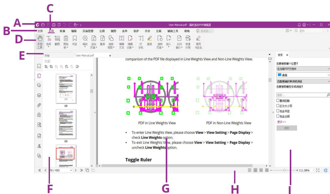
用户界面
