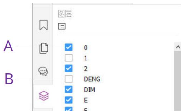
图层面板
